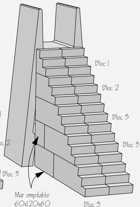
Composition escalier pour A400
